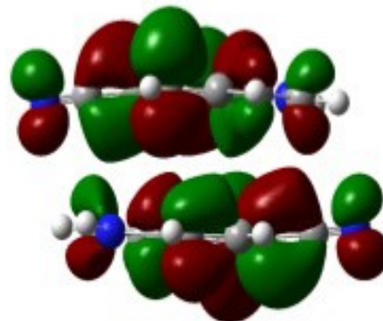
LUMO+1
