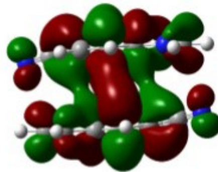
LUMO
