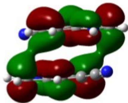
HOMO-1
