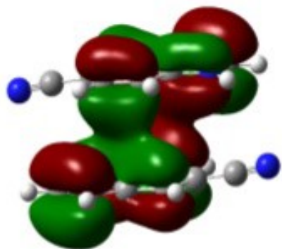
HOMO
