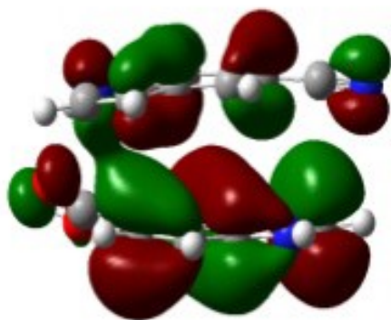
HOMO-1
