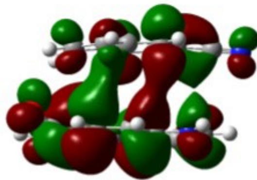
LUMO+1
