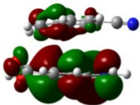
HOMO
