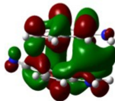
LUMO
