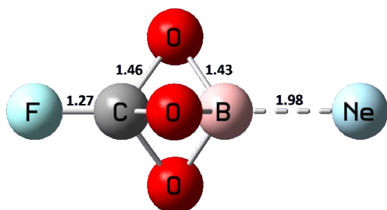
CBFO 3 Ne
