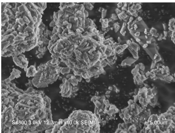
Figure S1 SEM images of SSZ-39, Cu-SSZ-39, Fe-Cu-SSZ-39
