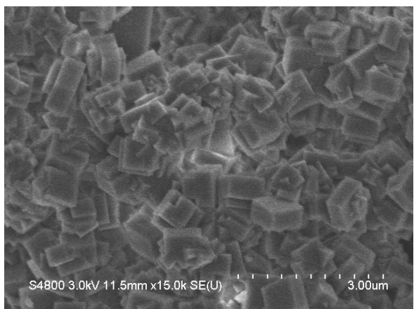
Figure S1 SEM images of SSZ-39, Cu-SSZ-39, Fe-Cu-SSZ-39
