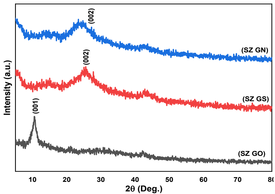
S1: XRD spectra of GO (SZ-GO), S-GO (SZ-GS), N-GO (SZ-GN) 1
