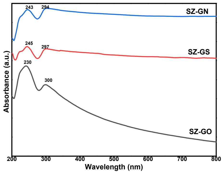
S3: UV-Visible spectra of SZ-GO, SZ-GS and SZ-GN
