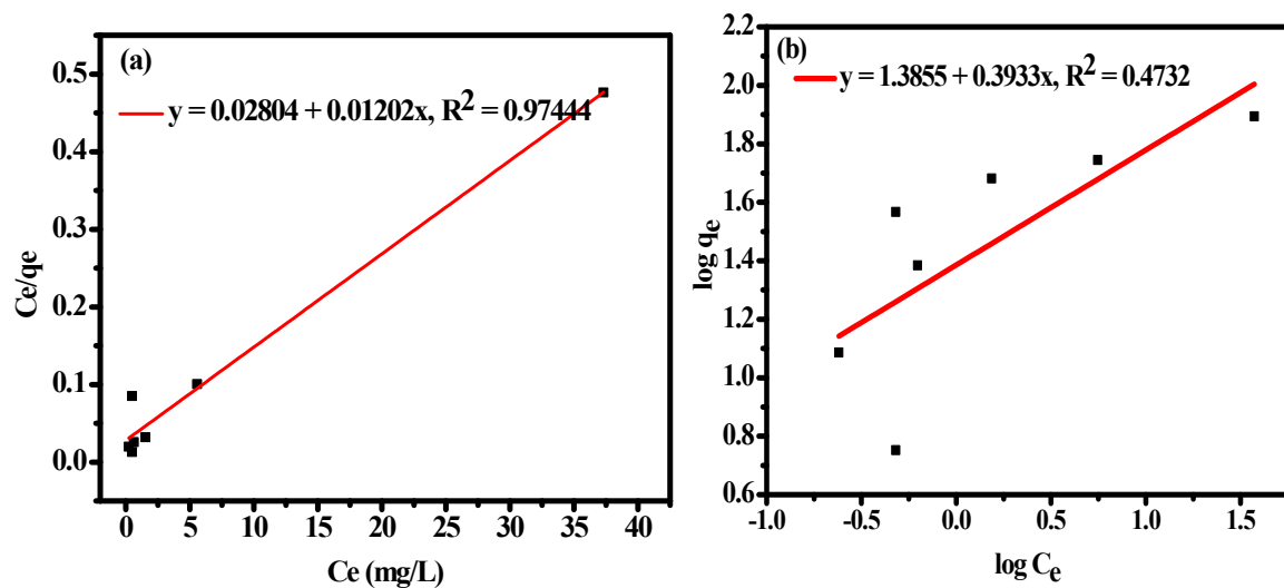
Fig. SI-2. (a) Langmuir isotherm and (b) Freundlich isotherm
