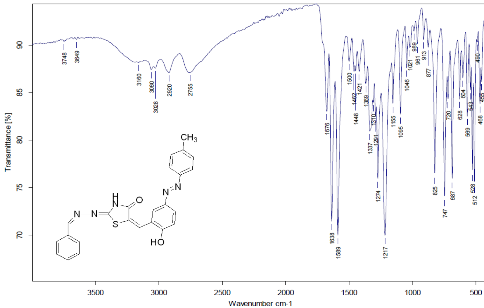
Figure. S5b A: IR spectrum of compound 5b(dye 4).
