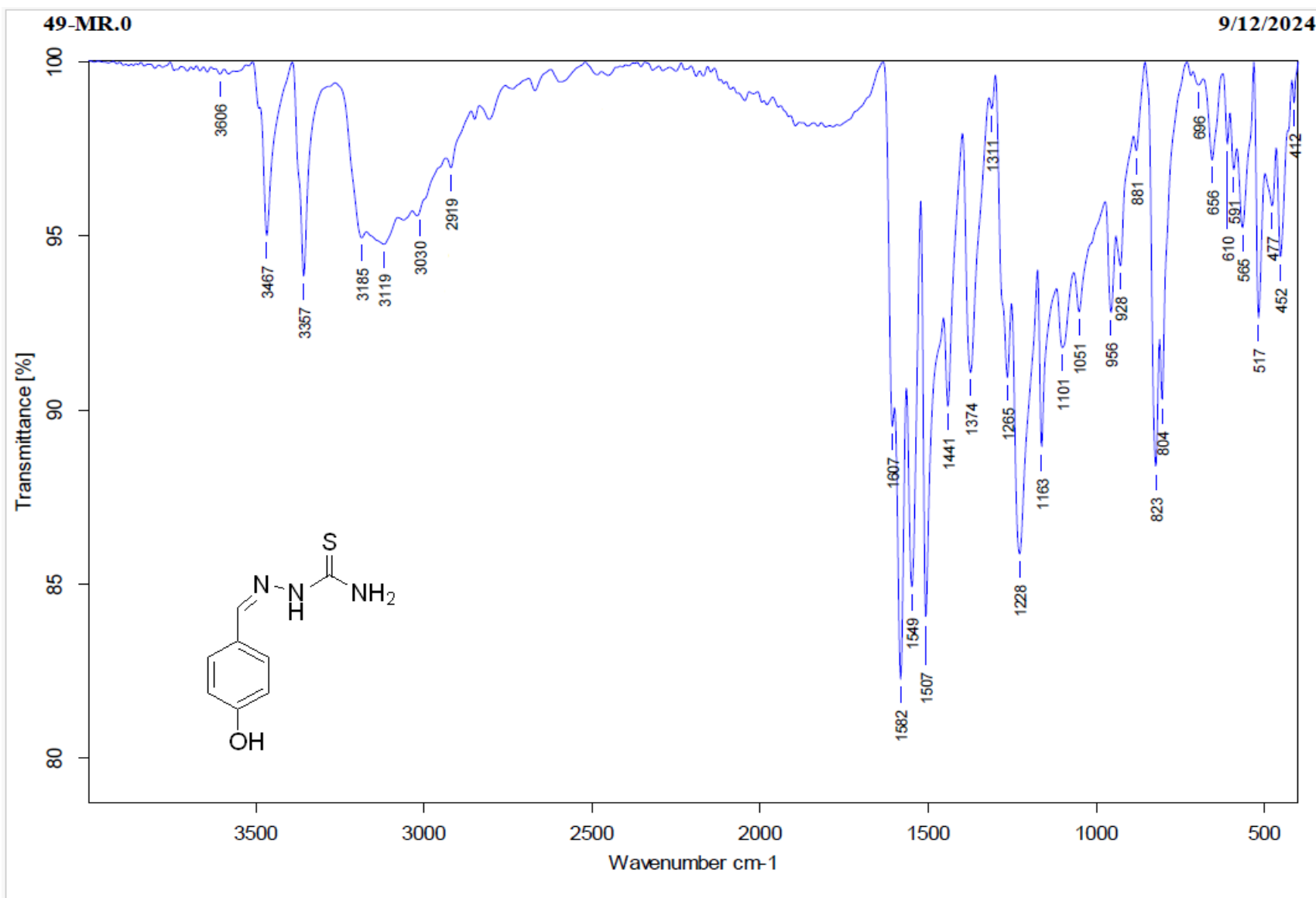
Figure. S1e A: IR spectrum of compound 1e
