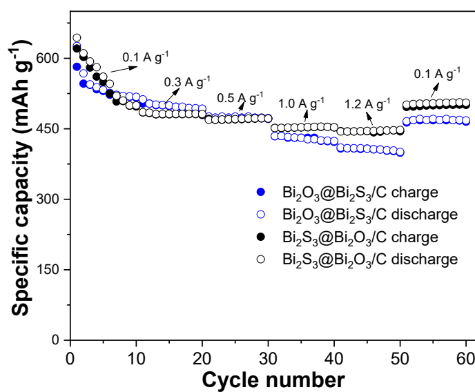
Fig. S3: Rate capability of Bi 2 S 3 @Bi 2 O 3 /C and Bi 2 O 3 @Bi 2 S 3 /C.
