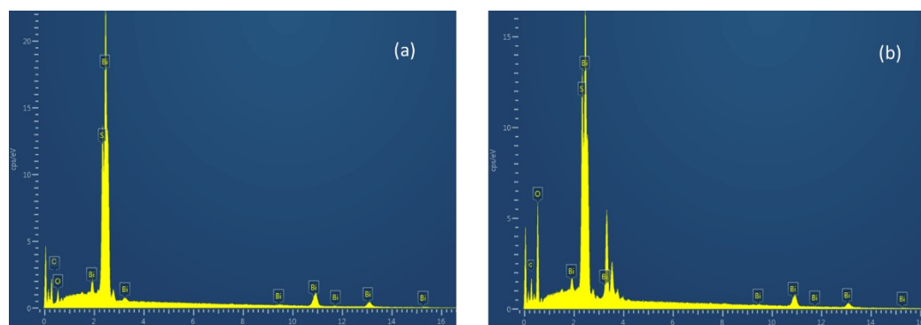
Fig. S2: EDS spectra of (a) Bi 2 S 3 @Bi 2 O 3 /C and (b) Bi 2 O 3 @Bi 2 S 3 /C.
