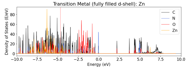
qmof-6c81e33:
