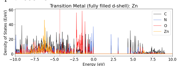
qmof-9931f8f:
