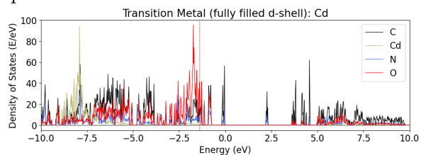
qmof-05305ab:
