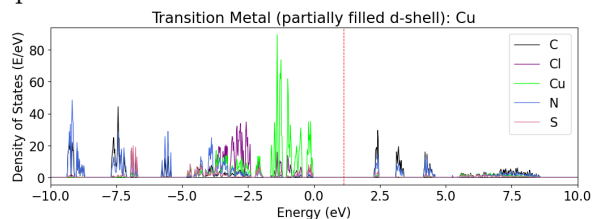
qmof-633815b:
