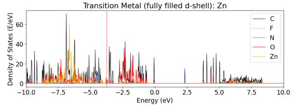
qmof-2446a3a:
