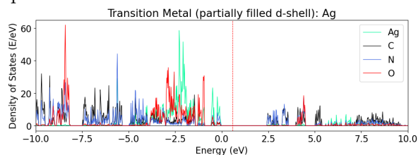
qmof-d689892:
