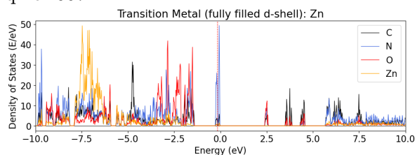
qmof-00744ff:
