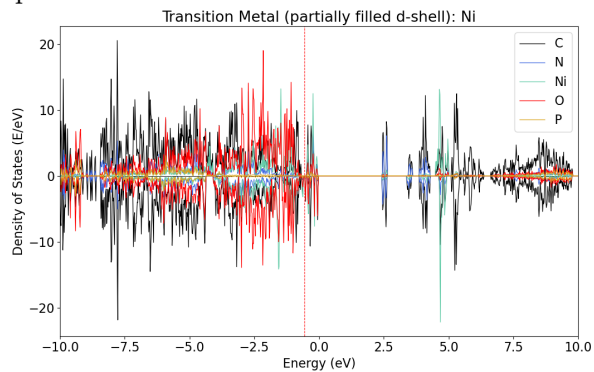
qmof-7e9d037:
