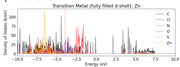
qmof-77e8bf6:
