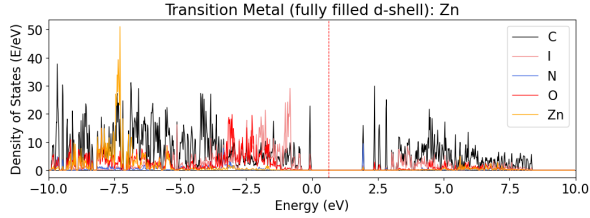
qmof-051793e:
