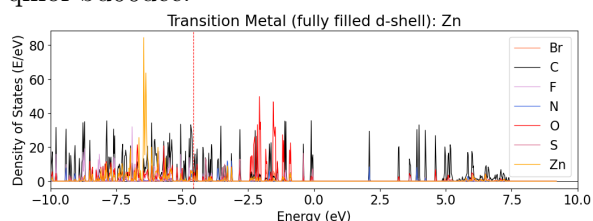
qmof-bd66dee:
