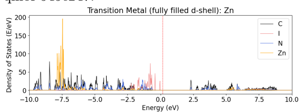
qmof-545c247:
