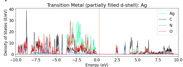
qmof-715f306:
