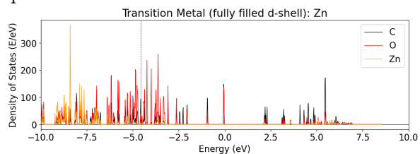
qmof-2cfb7a7:
