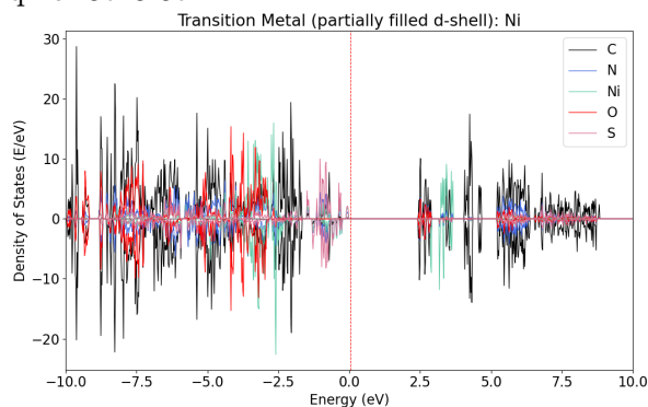
qmof-3c23f8c:
