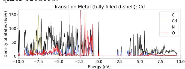
qmof-5108c60:
