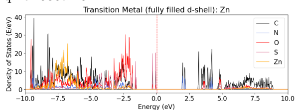
qmof-536a1f0:
