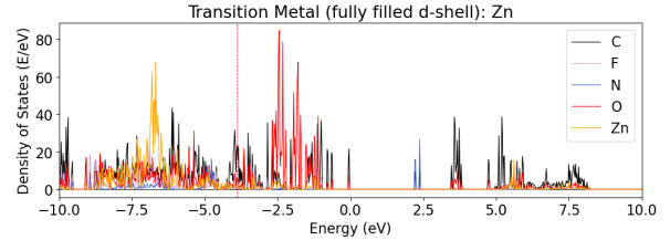
qmof-628ac43:
