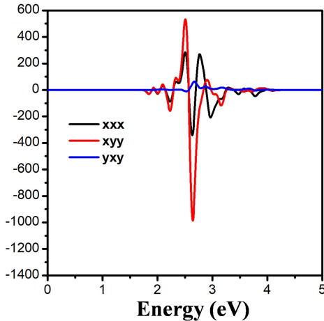
(d) MoS 2 /CrOCl, U = 4 eV
