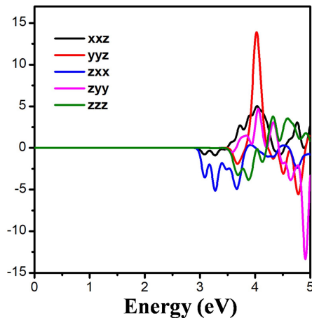
(d) MoS 2 /CrOCl, U = 4 eV
