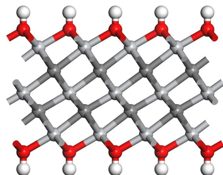
\text{Ti}_3\text{C}_2(\text{OH})_2
