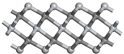
\text{Ti}_3\text{C}_2
