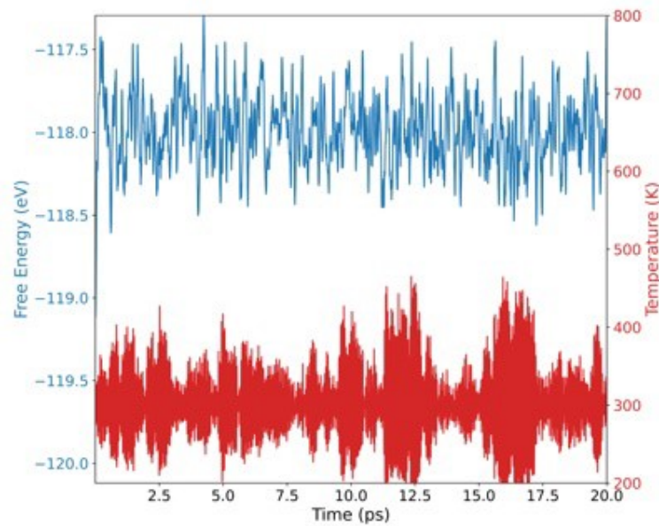
\text{In}_2\text{TeSe}
