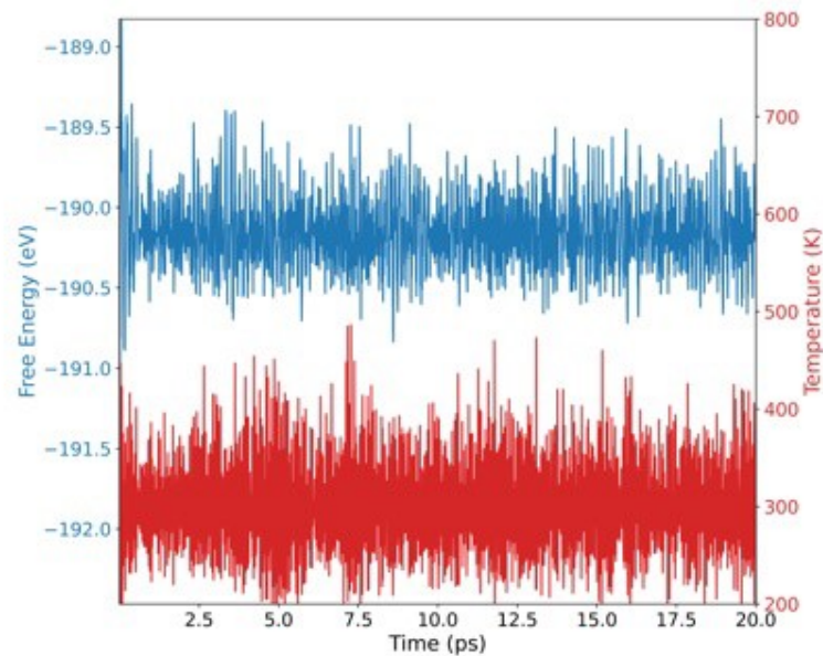
\text{B}_2\text{SeS}
