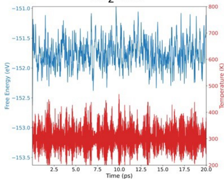
\text{AlSbAs}_2
