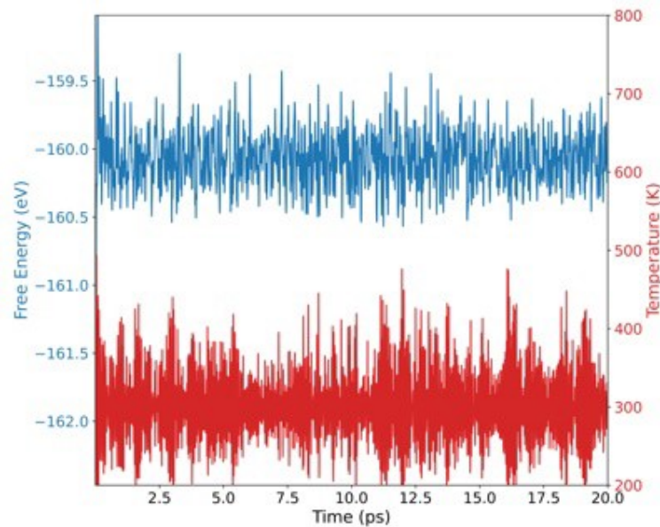
\text{Al}_2\text{SeS}
