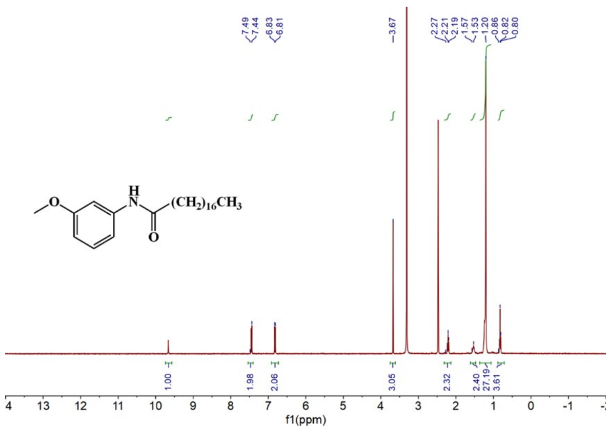
Figure S3. 1 H NMR spectrum of C1 (DMSO-d 6 ).
