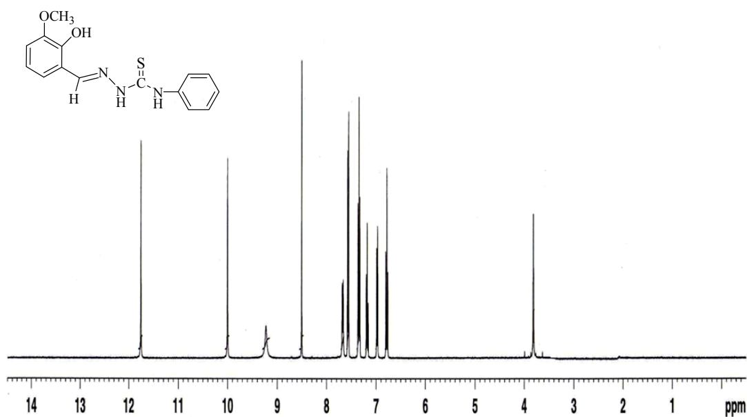
Fig. S7 ^1\text{H} -NMR spectrum of (\text{H}_2\text{L}^4)
