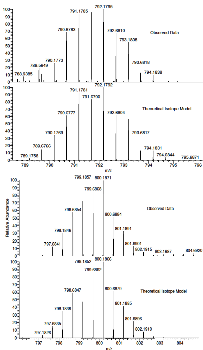
Fig. S1. Top : HR MS (ES + ) spectrum of [Ir(epqc) 2 (L 7 -Gd)](PF 6 ). Bottom : HR MS (ES + ) spectrum of [Ir(epqc) 2 (L 7 -Yb)](PF 6 ).
