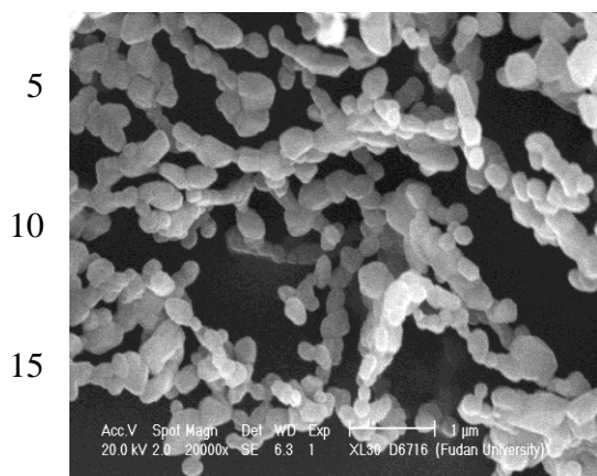
20 Fig..S1 SEM of LiMn 2 O 4 nanochain.
