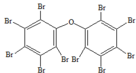
BDE209
