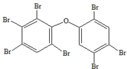
BDE 183
