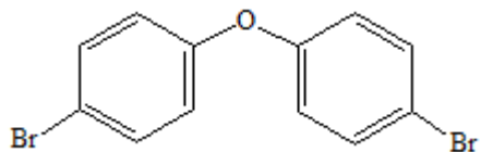
BDE 15
