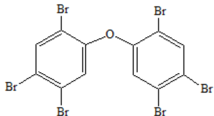
BDE 153
