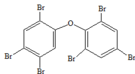
BDE 154
