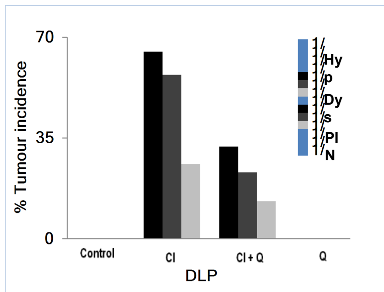
A) DLP
