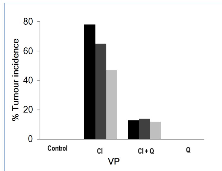
B) VP
