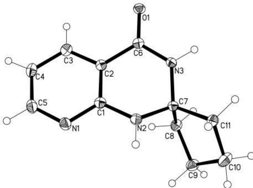
Fig. 1 ORTEP diagram of 3a
