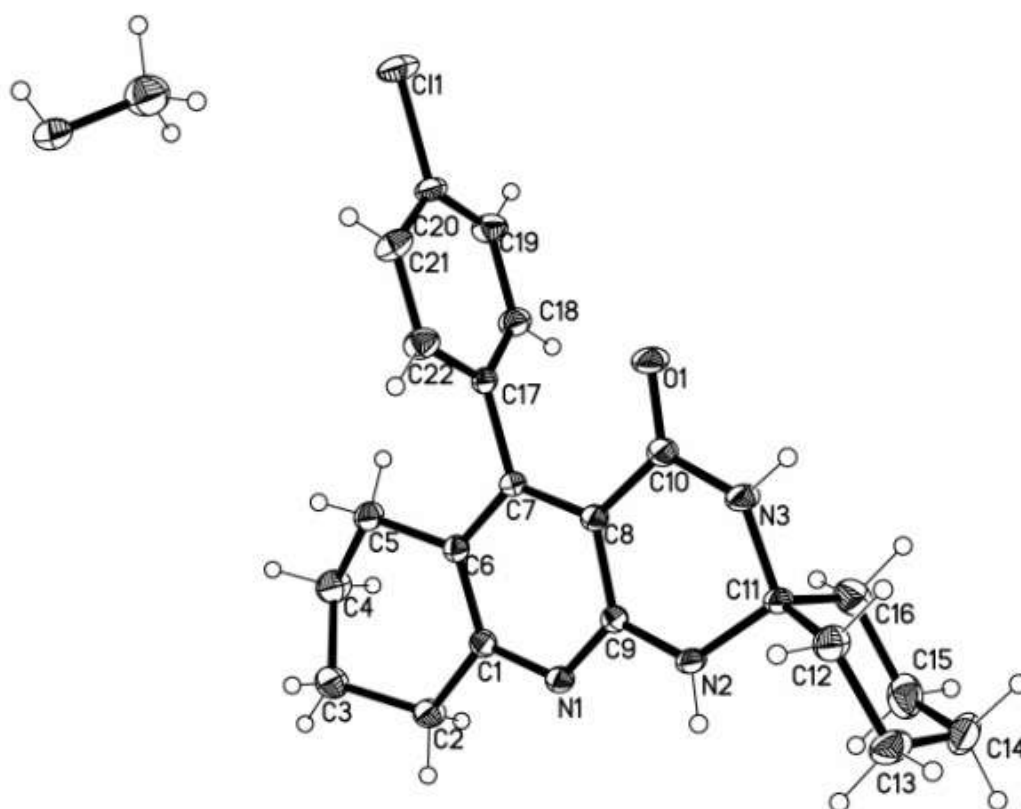
Fig. 3 ORTEP diagram of 4e
