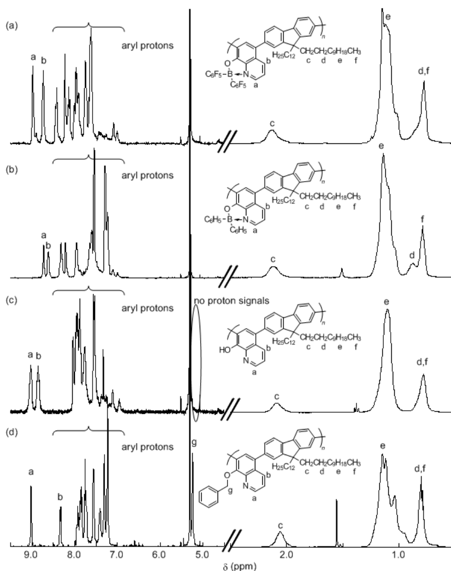
Fig. S1. 1 H NMR spectra of (a) poly4 , (b) poly3 , (c) poly2 , and (d) poly1 in CD 2 Cl 2 .
