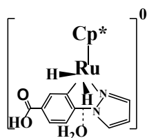
Ru-7'
