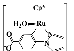
B Ru
