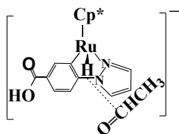
Ru-20
