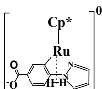
Ru-14
