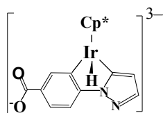
3-F Ir
