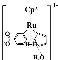
Ru-9
