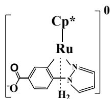
Ru-15
