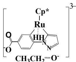
Ru-26
