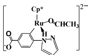
Ru-5
