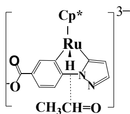
Ru-28
