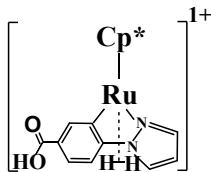
Ru-11
