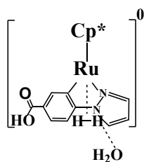
Ru-7
