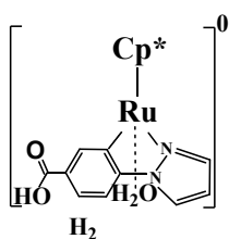
Ru-8
