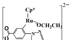
Ru-2
