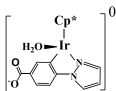
B Ir
