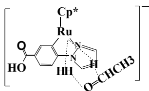
Ru-18
