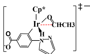
TS 9-10
