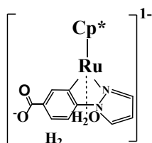
Ru-10
