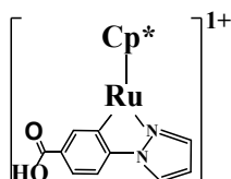
Ru-13
