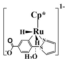
Ru-9'
