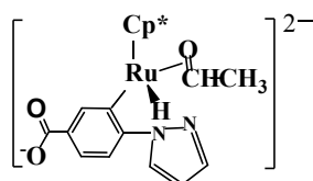
Ru-4
