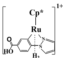
Ru-12
