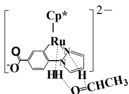
Ru-22
