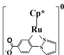
Ru-16
