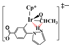
TS 8-9
