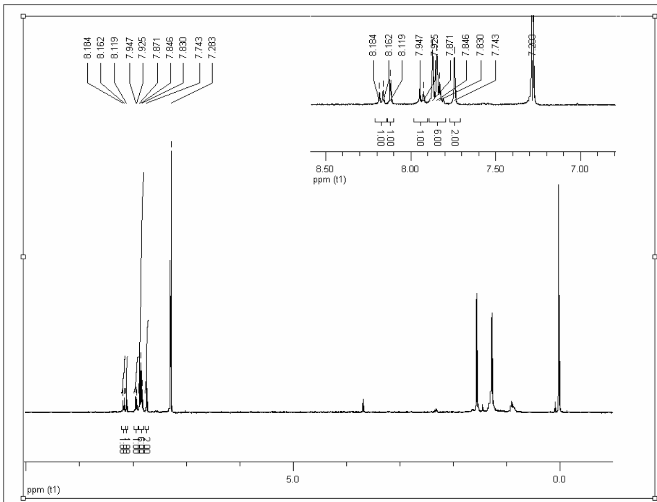
^1\text{H} NMR of 1,4 diethynylcorannulenebenzene (6)
