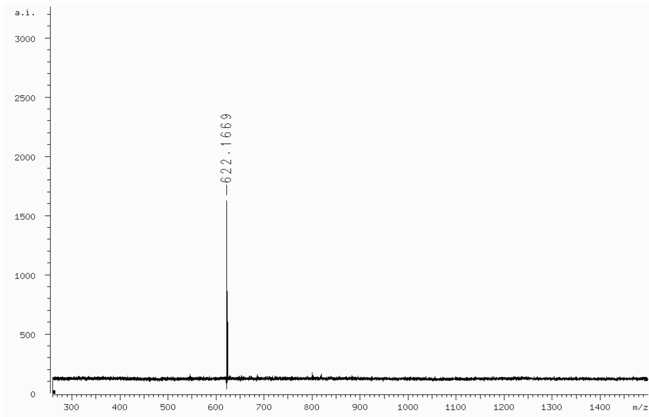
MALDI-TOF of 1,4 diethynylcorannulenebenzene (6)
