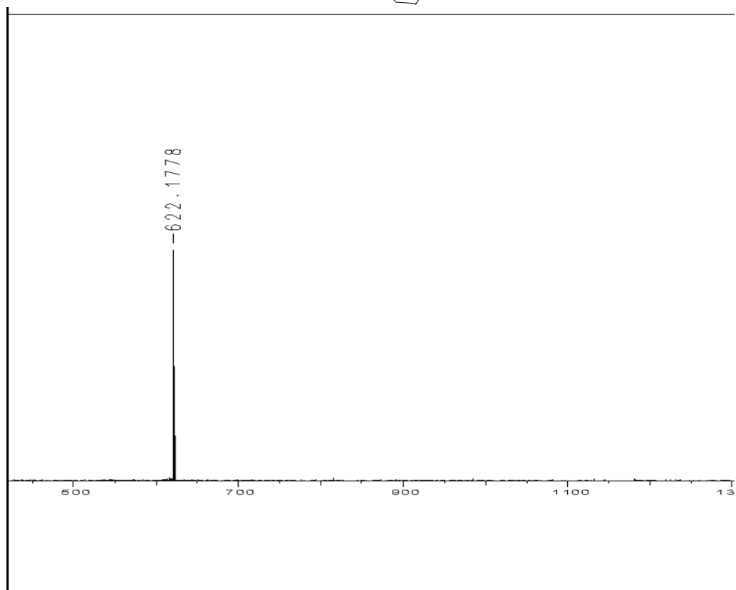
MALDI-TOF of 1,2 diethynylcorannulenebenzene ( 5 )
