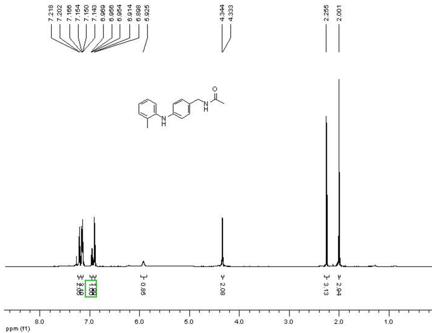
1 H-NMR 4b
