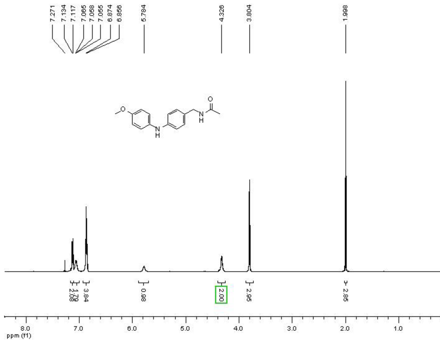
1 H-NMR 4c
