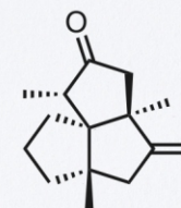
18 HMBC
