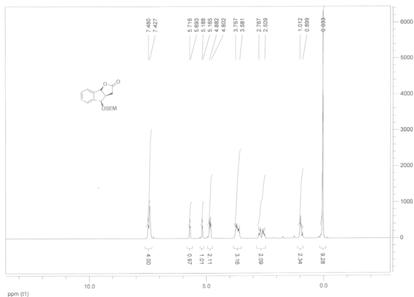
(3a S *,4 R *,8b S *)-4-((2-(trimethylsilyl)ethoxy)methoxy)-3,3a,4,8b-tetrahydro-2 H -indeno[1,2- b ]furan-2-one ( 15b )
