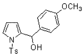
(4-Methoxyphenyl)-[1-( p -tolylsulfonyl)pyrrole-2-yl]methanol ( 16 )
