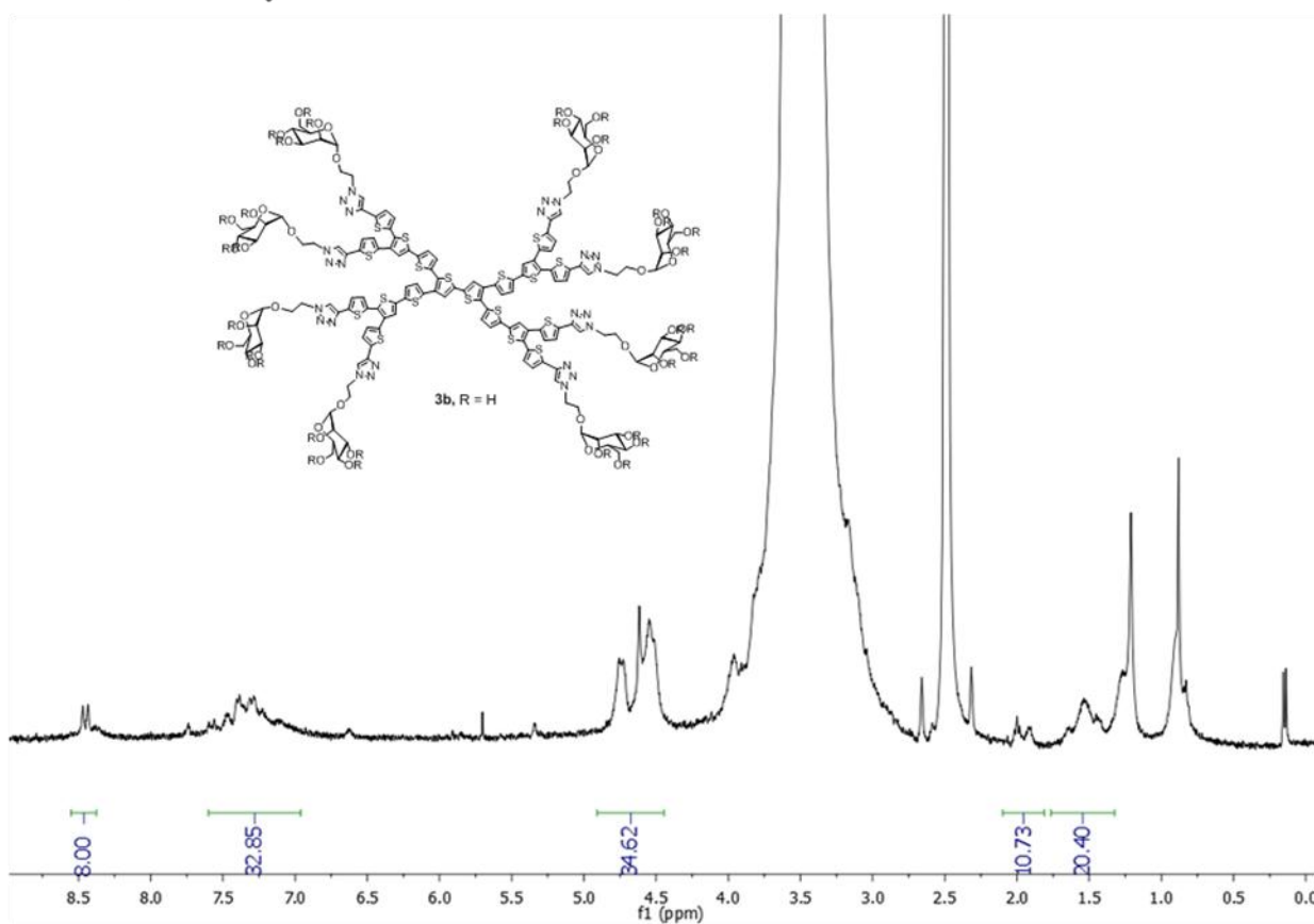
^1\text{H-NMR} , \text{DMSO-d}_6 , 3b
