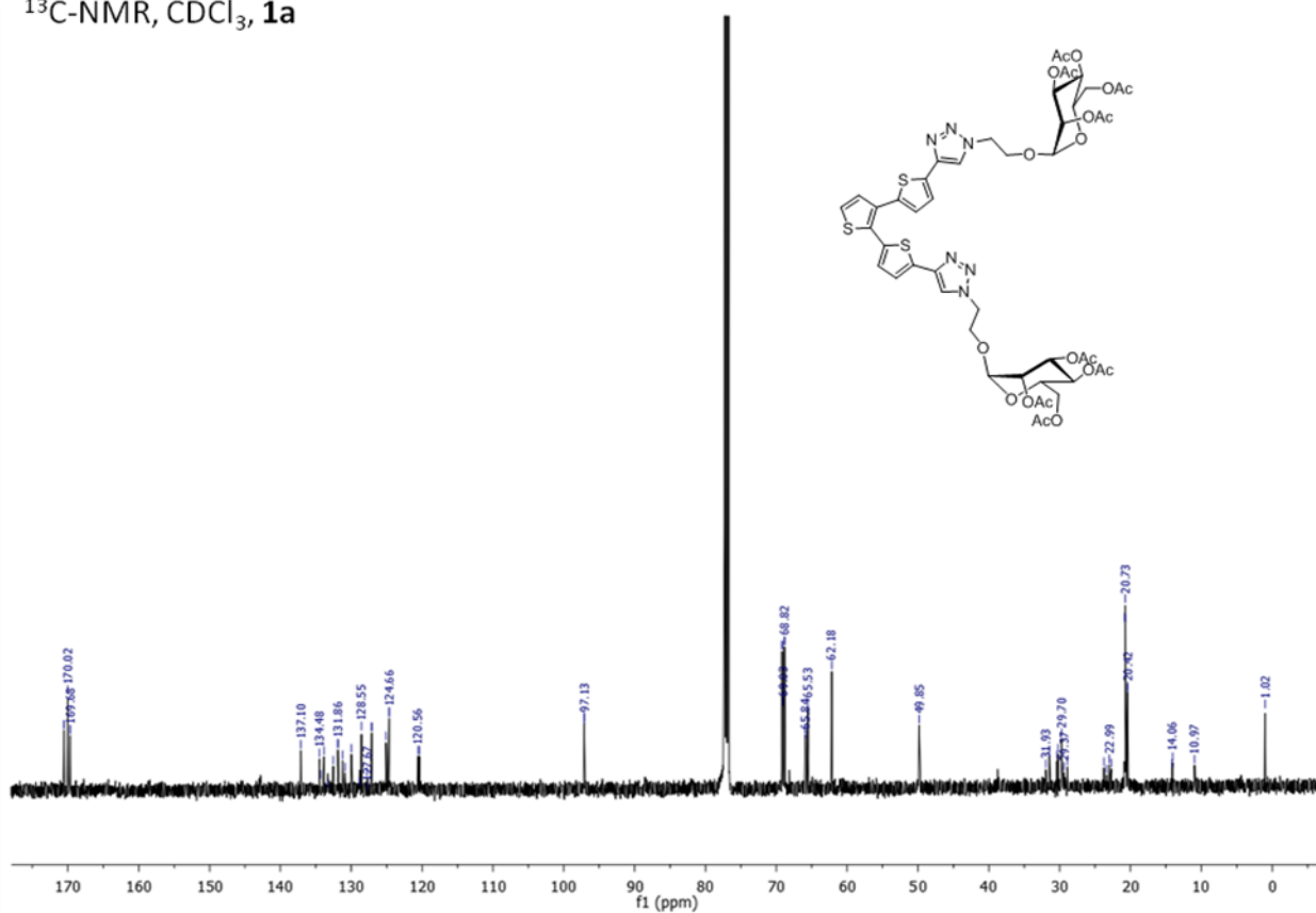
^{13}\text{C-NMR} , \text{CDCl}_3 , 1a
