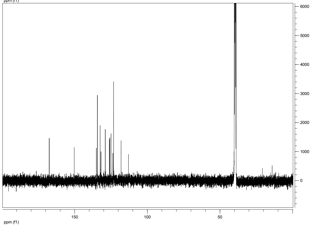
Compound 7e
