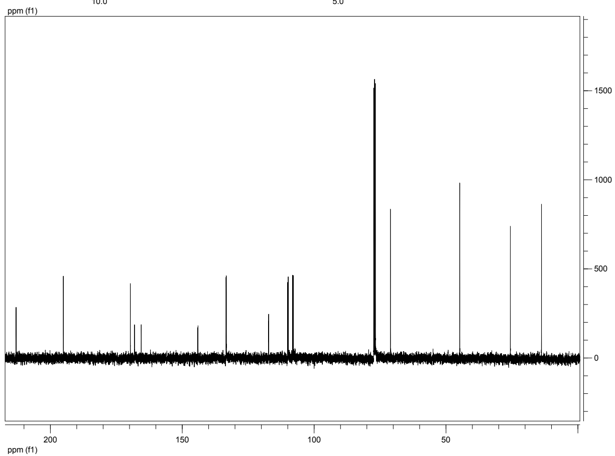
Compound 15e
