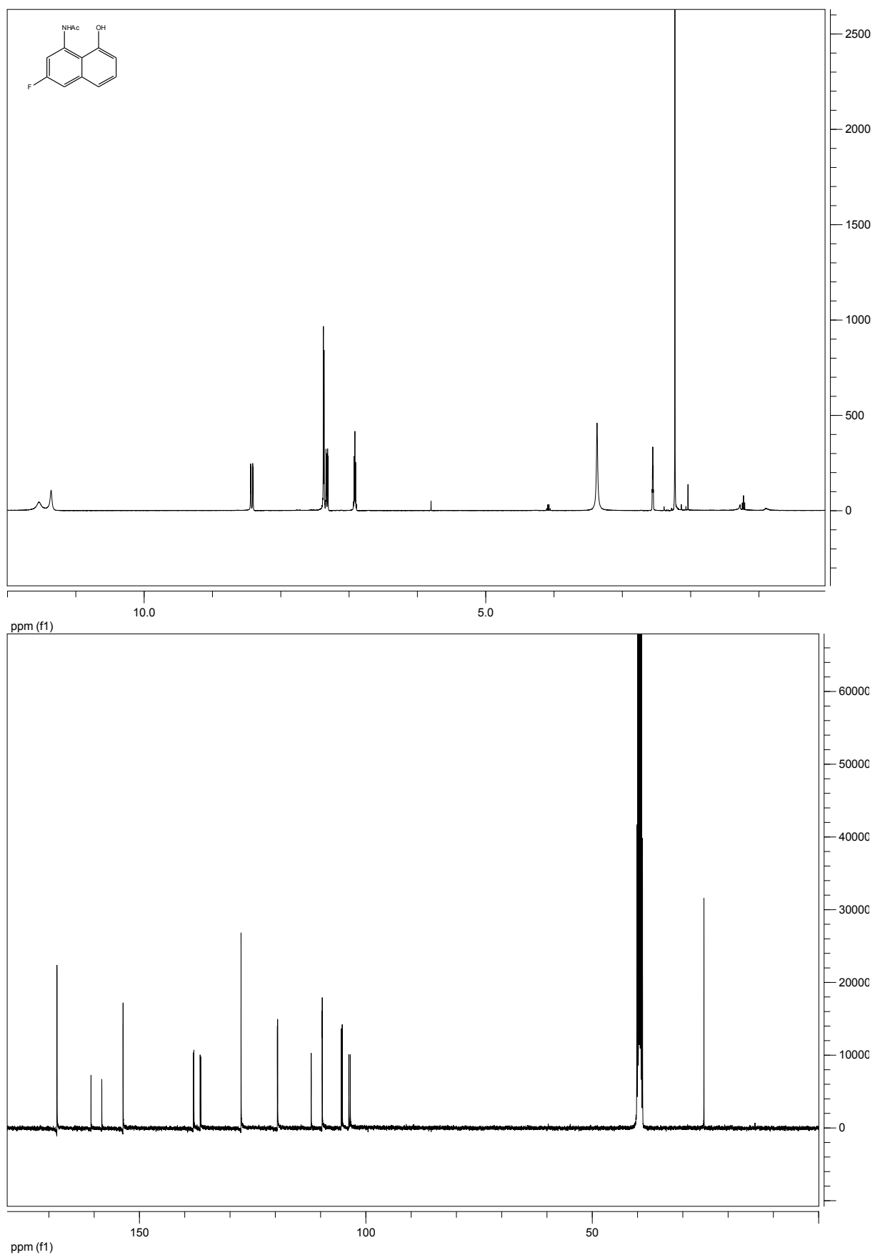
Compound 18e
