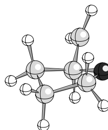
(2-furanyl)methyl
