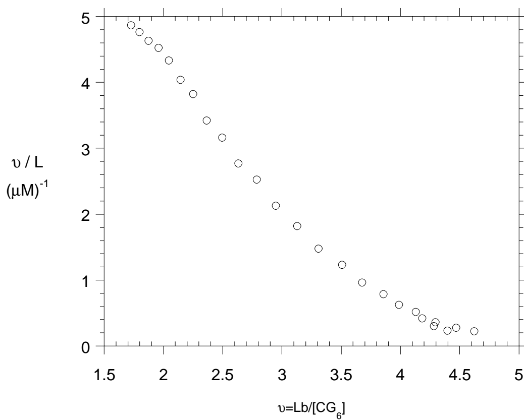
SSS ( \Delta ) + (CG) 6 McGhee-von Hippel plot
