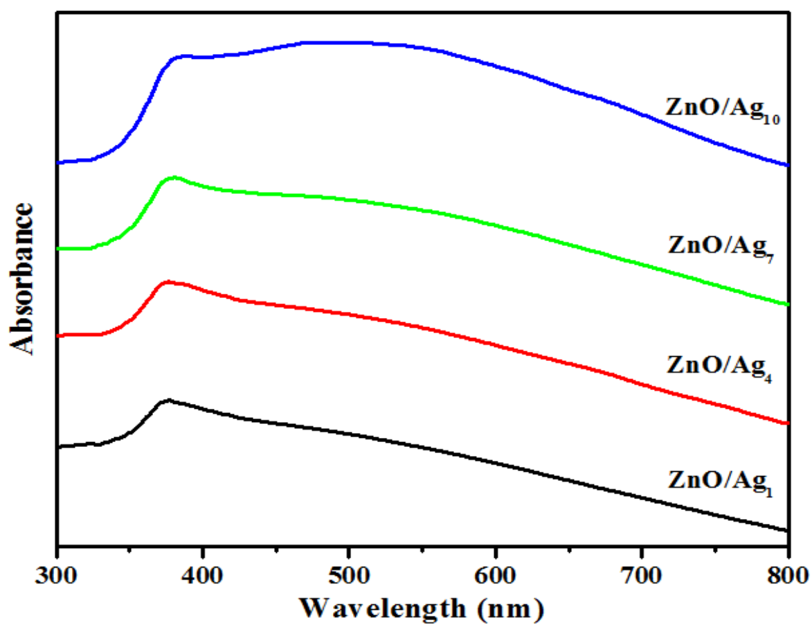
Fig. S2 UV-Visible spectra of ZnO/Ag 1 , ZnO/Ag 4 , ZnO/Ag 7 and ZnO/Ag 10 .
