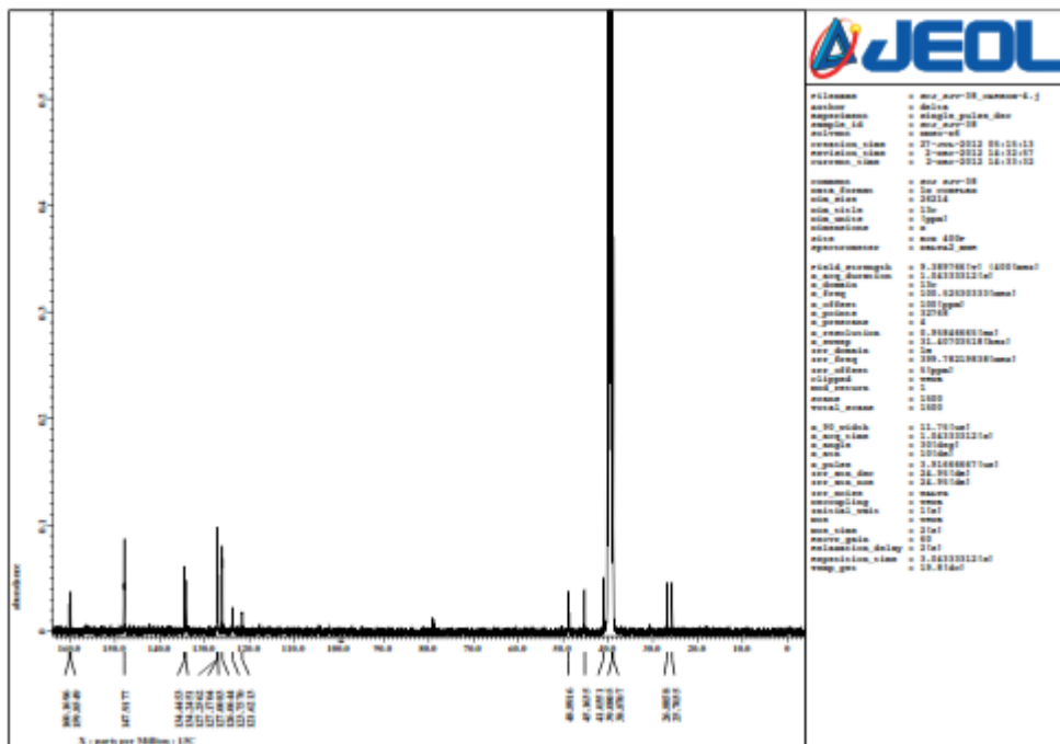
4-(4-(4-(Isoindolin-1,3-dion-2-ylmethyl)-1H-1,2,3-triazol-1-yl)butyloxy)quinazoline (1h)
