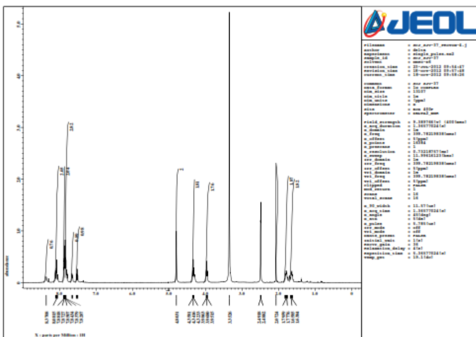
4-(4-(4-(Isoindolin-1,3-dion-2-ylmethyl)-1H-1,2,3-triazol-1-yl)butyloxy)quinazoline (1h)
