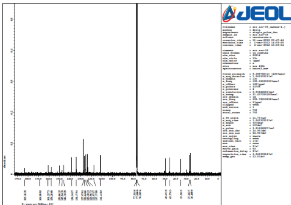
4-(6-(4-(1-Hydroxymethyl)-1 H -1,2,3-triazol-1-yl)hexyloxy)quinazoline (2b)
