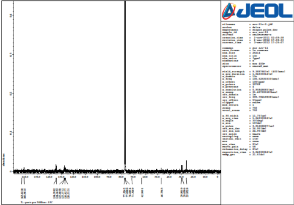
4-(6-(4-(Isoindolin-1,3-dion-2-ylmethyl)-1H-1,2,3-triazol-1-yl)hexyloxy) quinazoline (2h)
