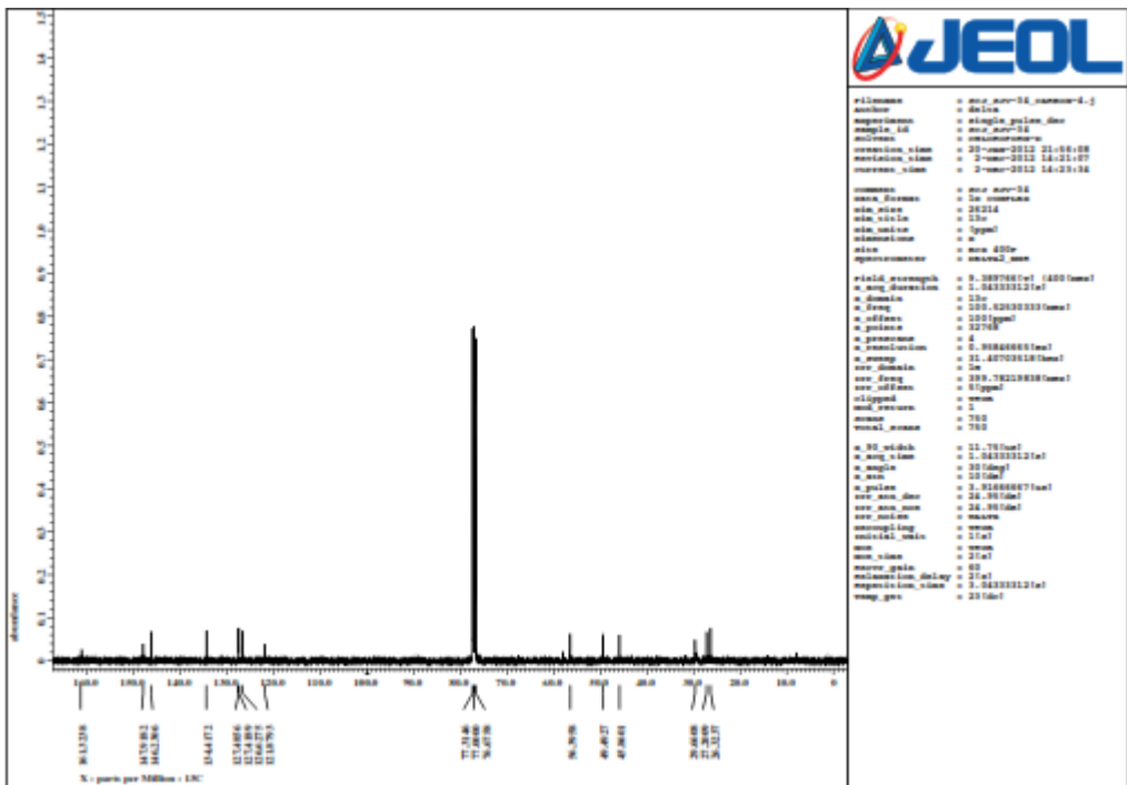
4-(4-(4-(1-Hydroxyethyl)-1 H -1,2,3-triazol-1-yl) butyloxy)quinazoline (1c)
