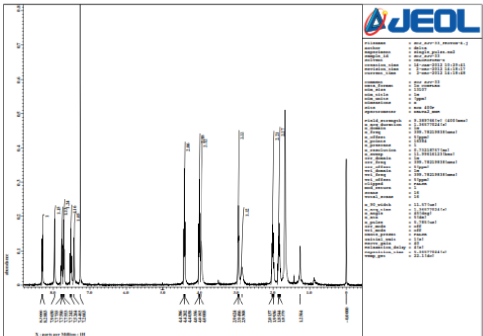
4-(4-(4-(1-Hydroxyethyl)-1 H -1,2,3-triazol-1-yl) butyloxy)quinazoline (1c)
