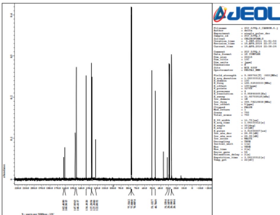
4-(4-(4-(1-Hydroxymethyl)-1 H -1,2,3-triazol-1-yl)butyloxy)quinazoline (1b)
