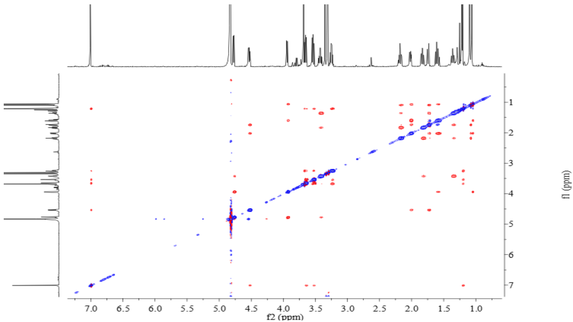
Lanceolatin G (7)
