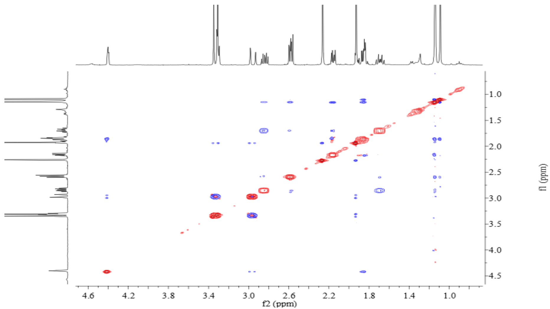
Lanceolatin D (4)
