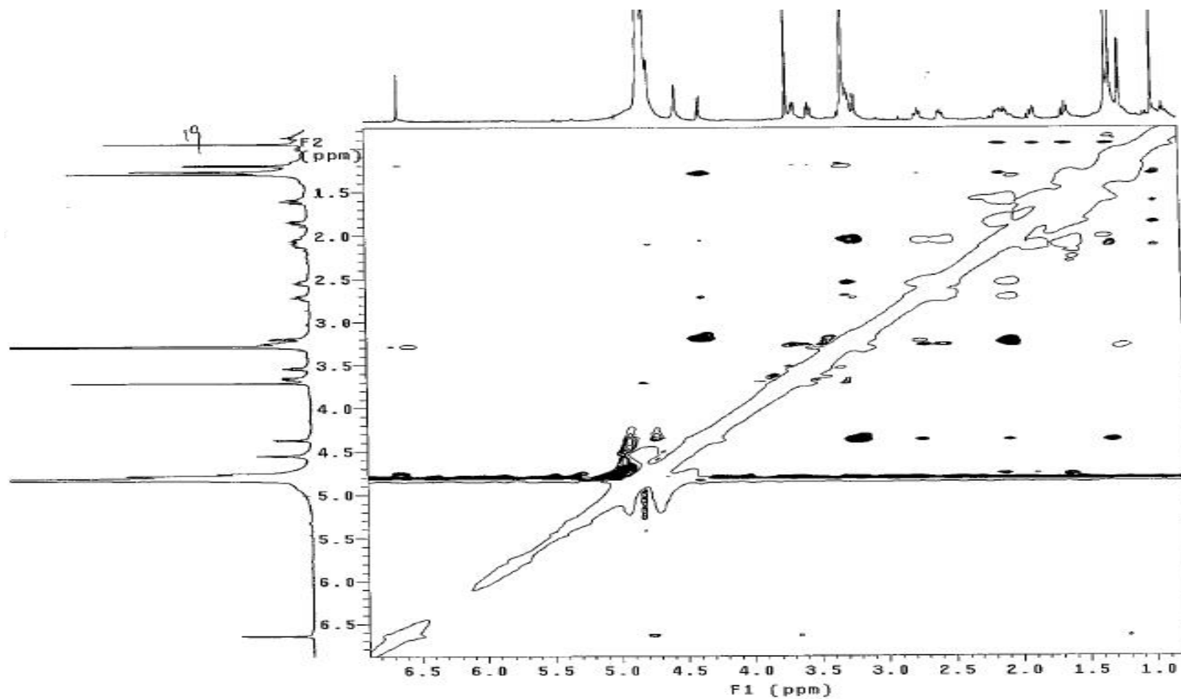
Lanceolatin E (5)
