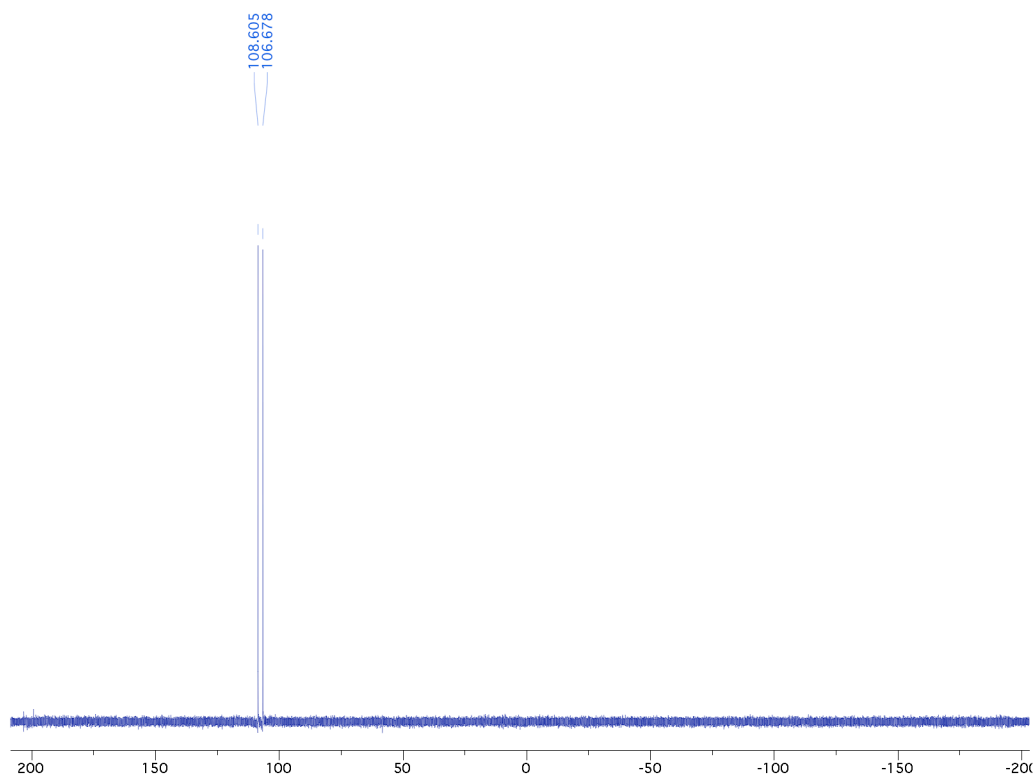
^{31}\text{P} -NMR Rh(cod)Cl•T1
