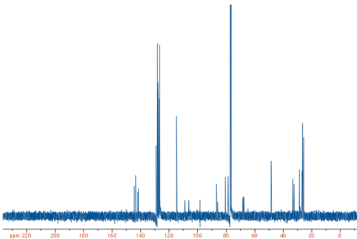
^{13}\text{C-NMR} \text{Rh(cod)Cl}\cdot\text{T1}
