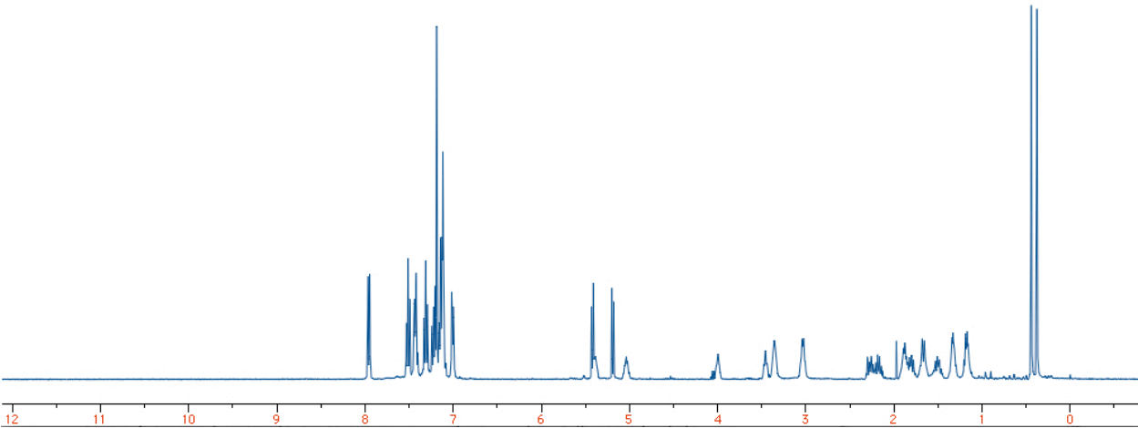
1 H-NMR Rh(cod)Cl• T1
