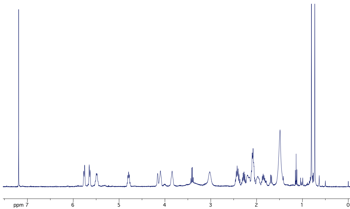
^1\text{H} NMR of Rh(cod)Cl·CKphos
