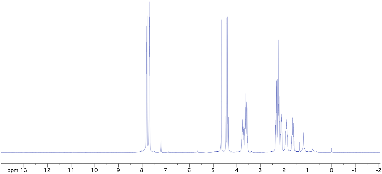
1 H NMR
