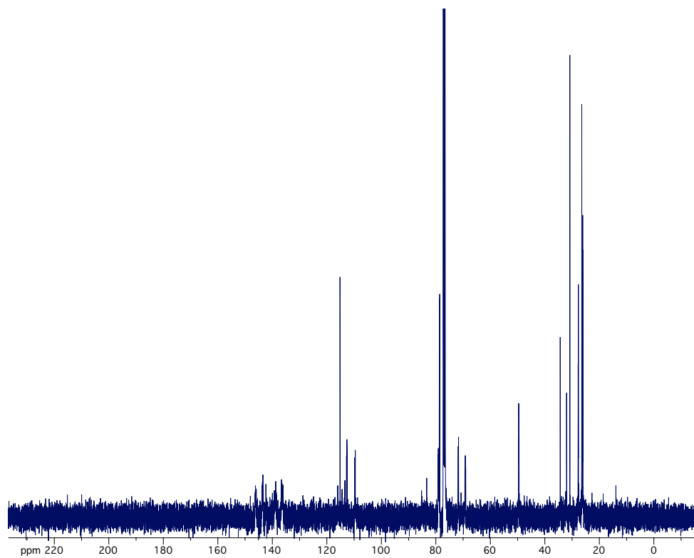
^{13}\text{C} NMR of Rh(cod)Cl·CKphos
