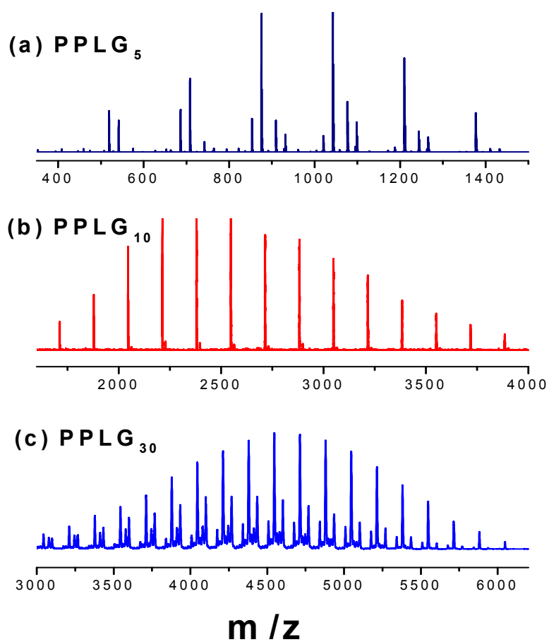
Figure S4: MALDI-TOF MS spectra of (a) PPLG 5 , (b) PPLG 10 and (c) PPLG 30
