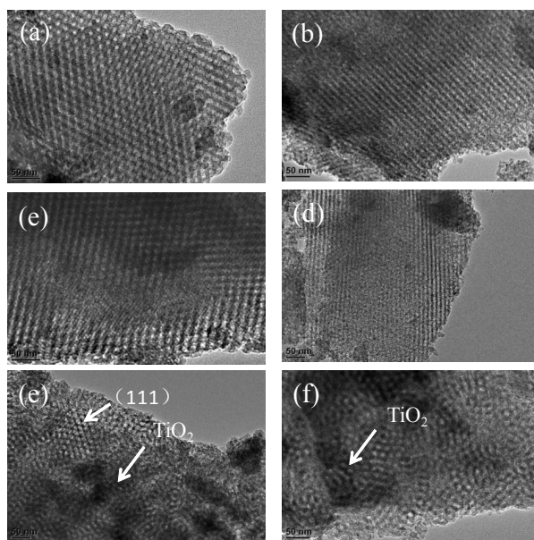
Fig. S1. TEM images of different samples (a) FDU-12 (b) ST-40 (c) ST-20 (d) ST-10 (d) ST-5 (e) ST-2.5.
