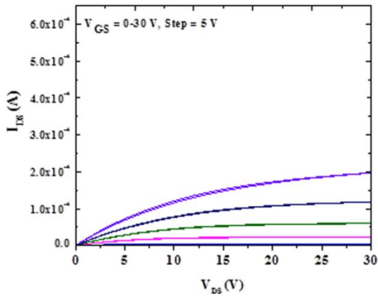
7 % O_2/Ar -a-BIZO TFT
