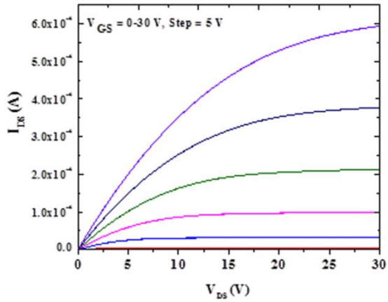
3 % O_2/Ar -a-BIZO TFT
