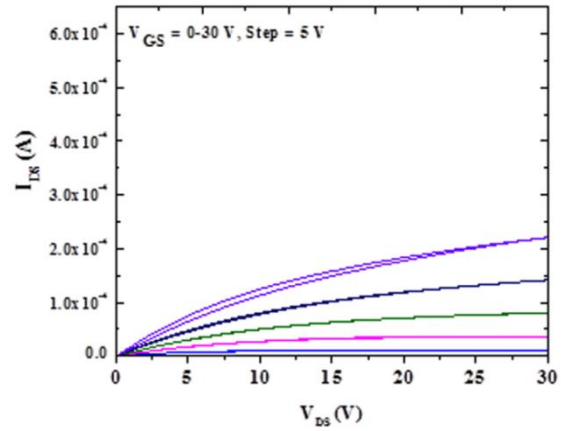
9 % O_2/Ar -a-BIZO TFT
