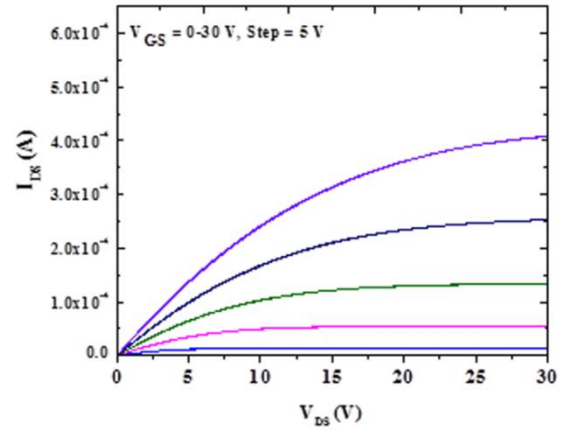
5 % O_2/Ar -a-BIZO TFT
